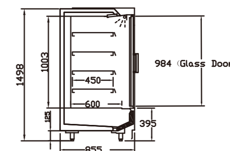
MenEco 腾跃系列 1.5 米半高玻璃门冷藏立柜
