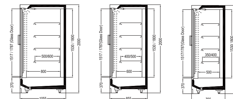
MenEco 腾跃系列玻璃门冷藏立柜
