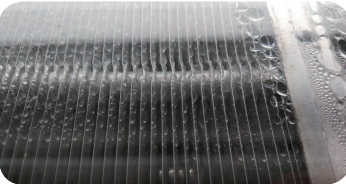
灵境无霜午餐柜： 标准工况下只有水珠附着于蒸发器， 无凝霜，没有化霜过程
